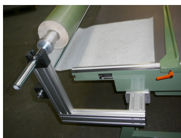
Despositivo desbobinator
